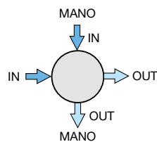
Anschlusschema
